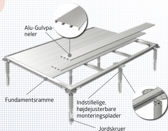
Fig. jordskruefundament
